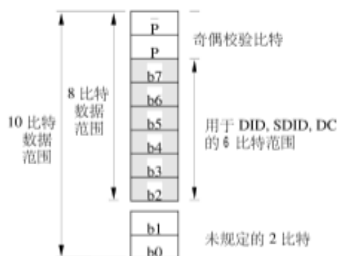
图 A2 8 比特 DI D、SDI D、DC 应用的编码范围
