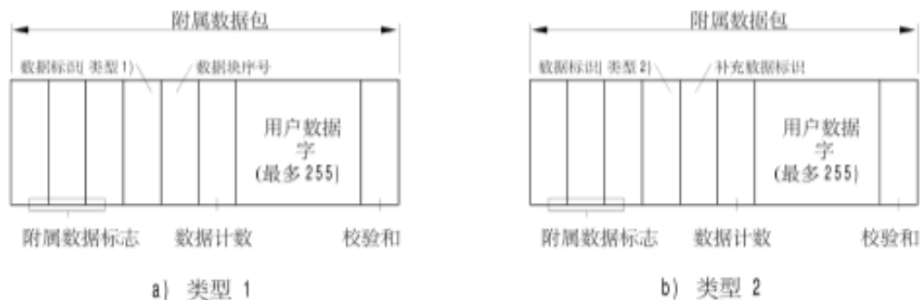
图 1 附属数据包类型
