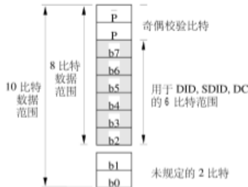
图 A2 8 比特 DI D、SDI D、DC 应用的编码范围
