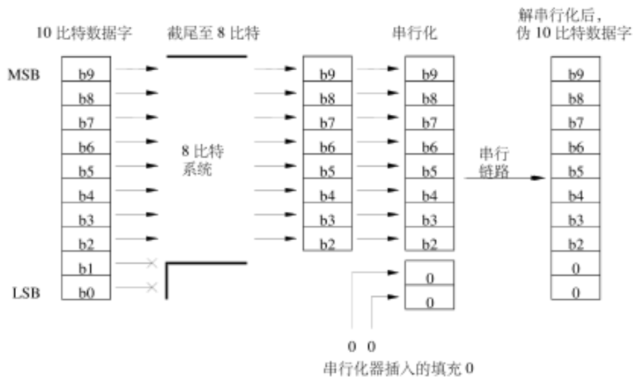
图 A1 数据字截尾的掺杂
